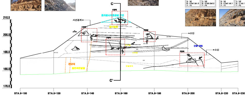
【그림 36.15】 상주절토36 검토대상 비탈면구간
