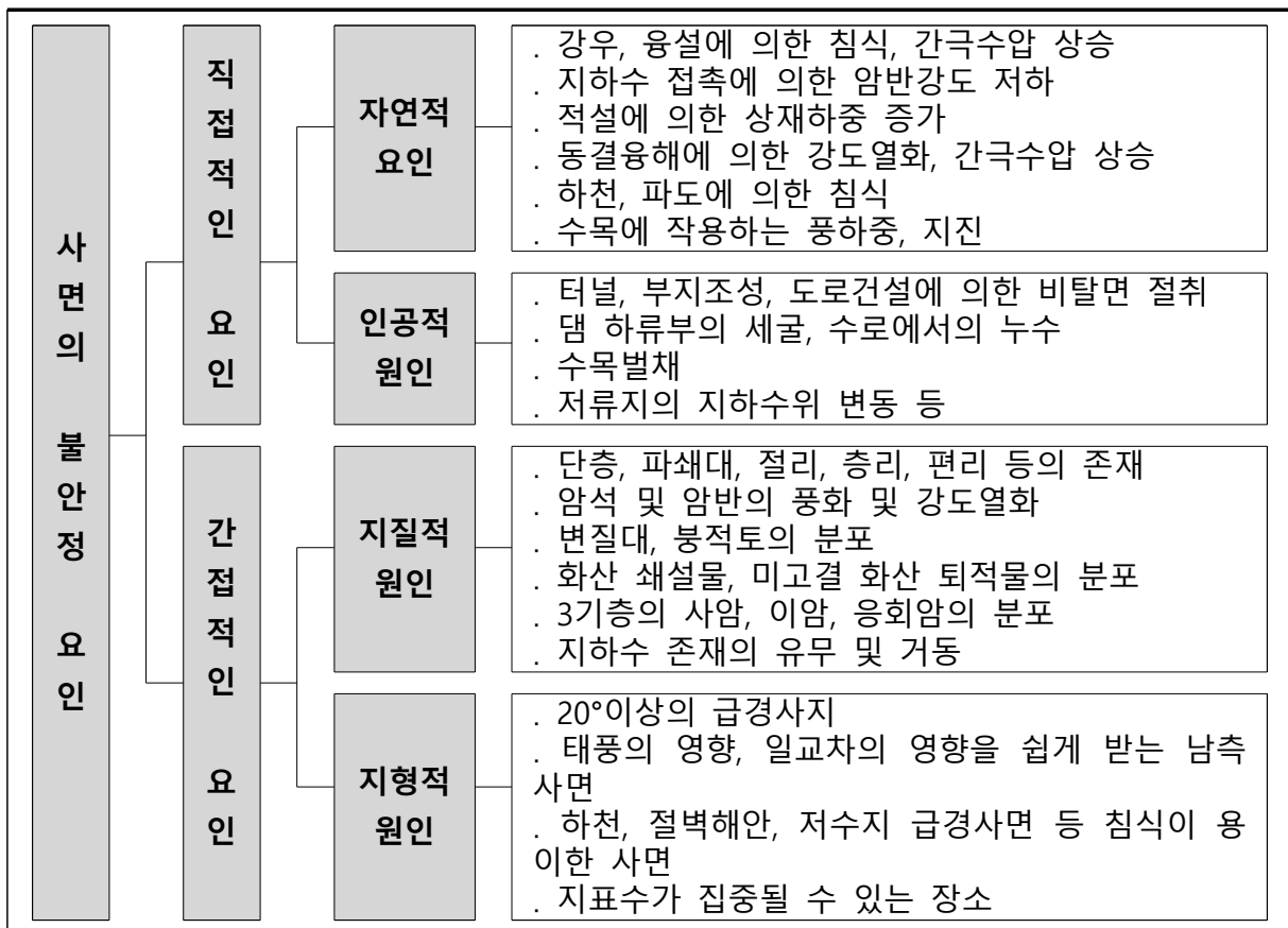
【그림 36.6】 구조안전성능 평가과정
